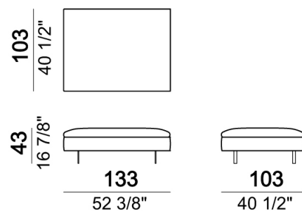
Pouf
