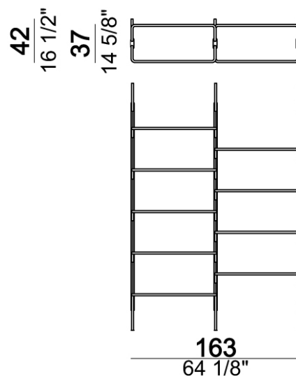
Libreria a parete "3-01W" (3 montanti W + 1 ripiano a terra 80T + 8 ripiani da 80 cm + 1 piede F).
