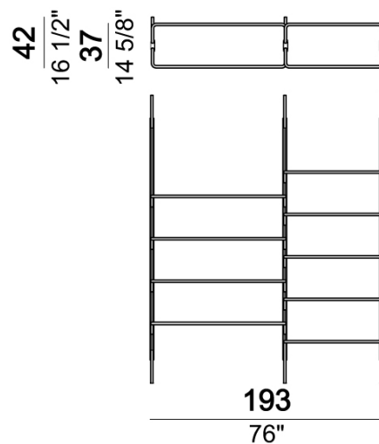
Libreria a parete "3-05W" (3 montanti W + 1 ripiano a terra 80T + 4 ripiani da 80 cm + 4 ripiani da 110 cm + 1 piede F).
