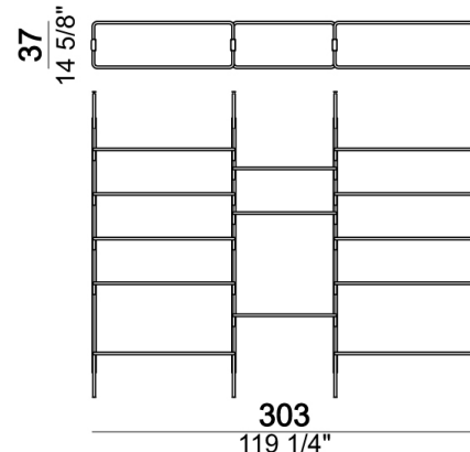
Libreria a soffitto "4-02C" (4 montanti C + 2 ripiani a terra 110T + 3 ripiani da 80 cm + 8 ripiani da 110 cm).
