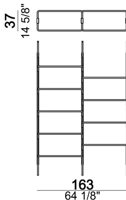
Libreria a parete "3-01W" (3 montanti W + 1 ripiano a terra 80T + 8 ripiani da 80 cm + 1 piede F).
