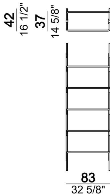
Libreria a parete "2-01W" (2 montanti W + 1 ripiano a terra 80T + 4 ripiani da 80 cm).
