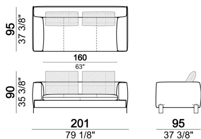
Divano / divano angolare SLIM
