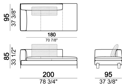
Laterale / laterale angolare dx o sx con pouf dx o sx
