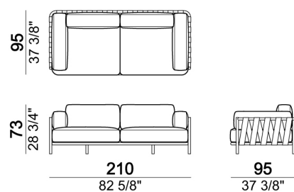
Divano
