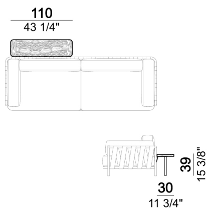
Cuscino bracciolo
