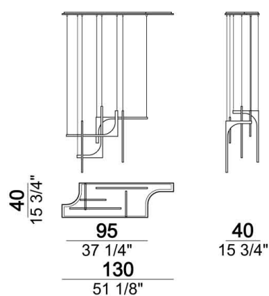
Lampada a sospensione con 5 luci
