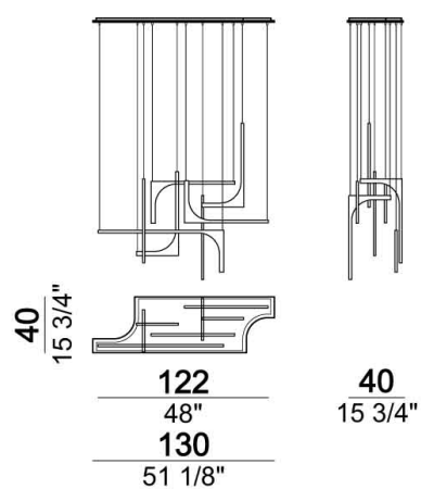
Lampada a sospensione con 7 luci
