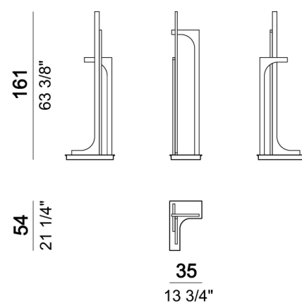
Lampada da terra a 3 luci
