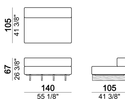
Seduta A3 + N.2 Schienali S1
