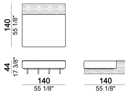
Seduta B2 + mensola
