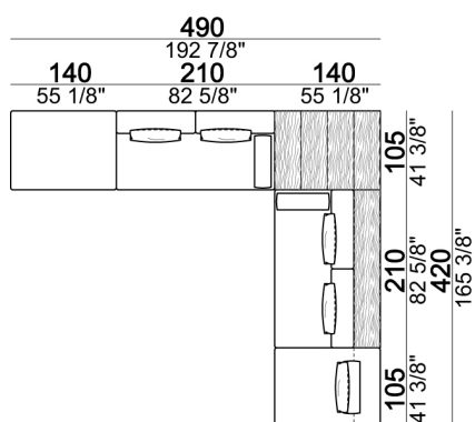
Seduta B3 + mensola + N.2 Schienali S1
